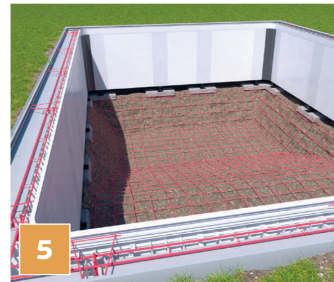
5 FERRAILLAGE DU FOND...
