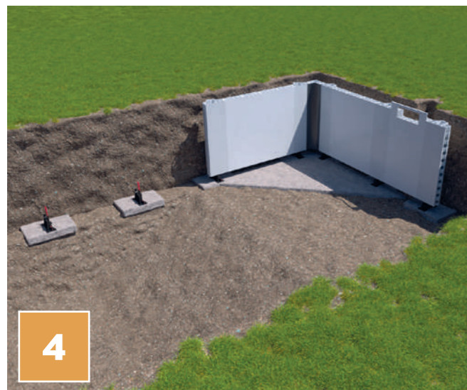
4 ALIGNEMENT DES STRUCTURES (Skimmer, projecteur... pré-installé en usine)
