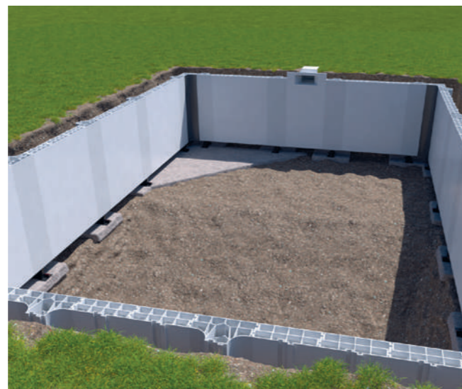
4 ALIGNEMENT DES STRUCTURES (Skimmer, projecteur... pré-installé en usine)
