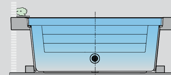
Installation autoportante avec supports de parois en acier laminé.
