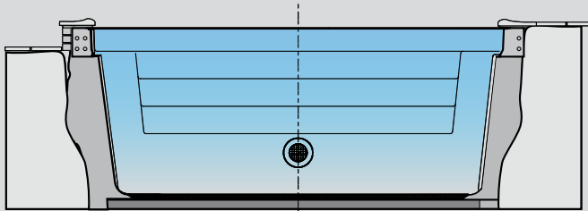
Installation sur une dalle en béton. Méthode pour les piscines extérieures.
