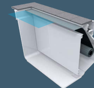
La niche prolonge la piscine d'environ 35 cm et raccourcit la longueur de nage d'env. 50 cm.
