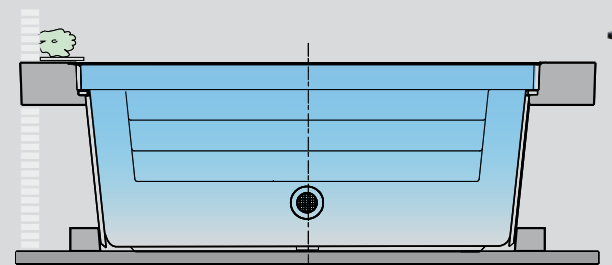
Installation autoportante avec supports de parois en acier laminé.
